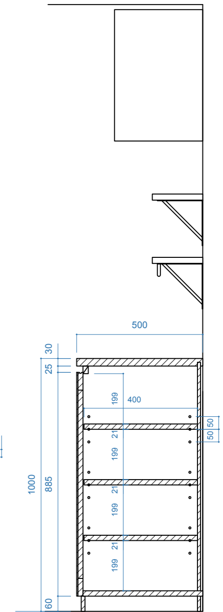
c断面図
